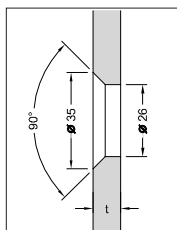
Glasbohrung für Senkzierschraube mit der Art.Nr. 200-0313
