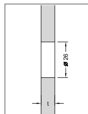
Glasbohrung für Blendschraube mit der Art.Nr. 200-0314
